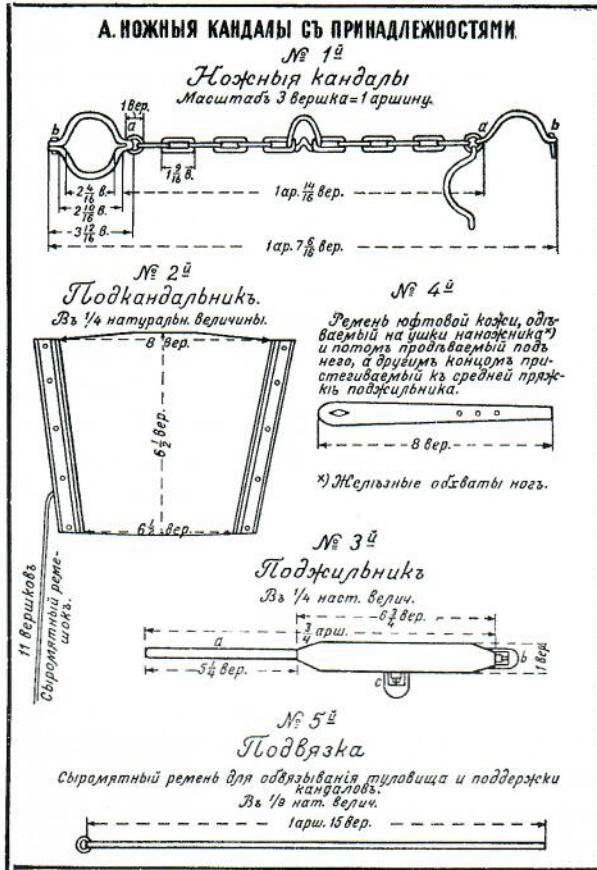
Чертеж кандалов
