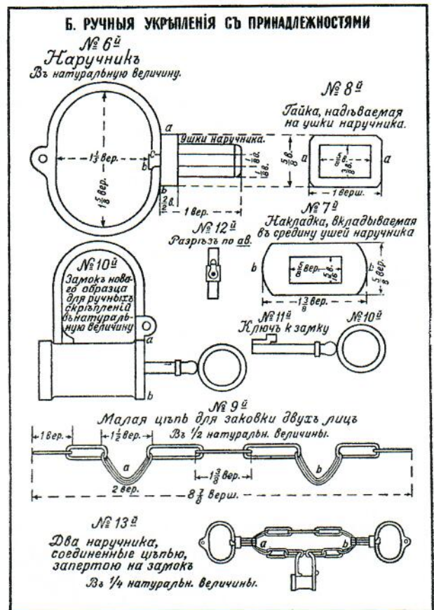
Чертеж кандалов
